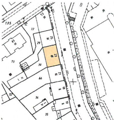
LAGEPLAN
